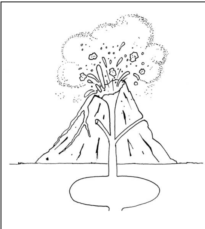
central conduit
