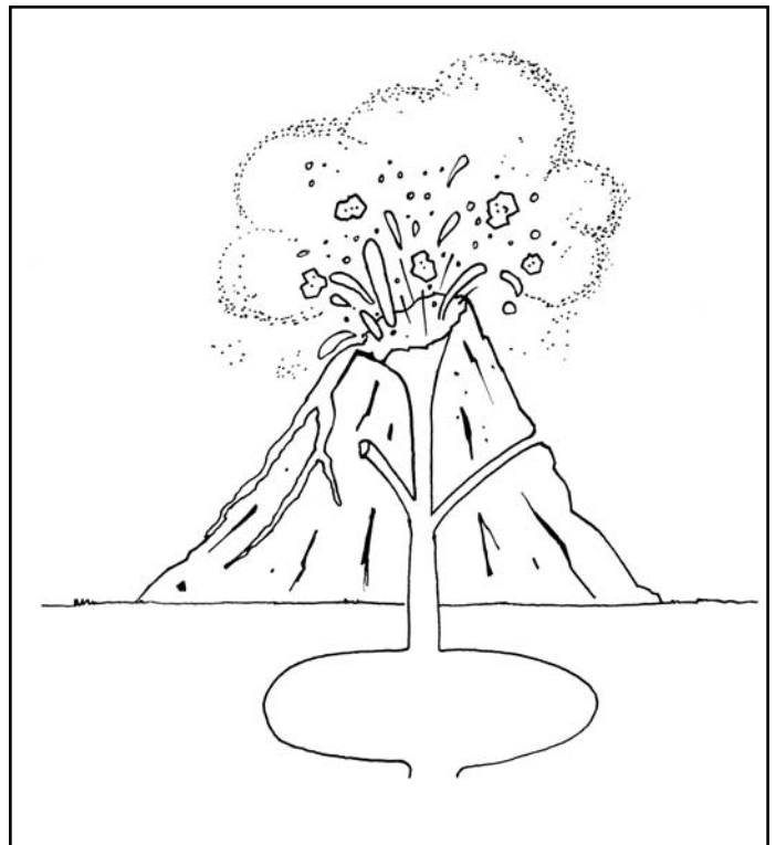
side conduit
